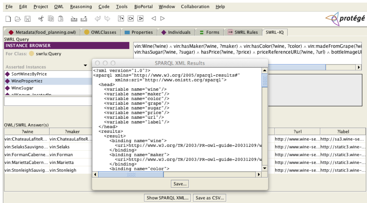
Fig. 11. Saving XML
